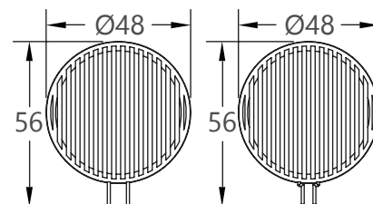
Base Type : GY6.35
